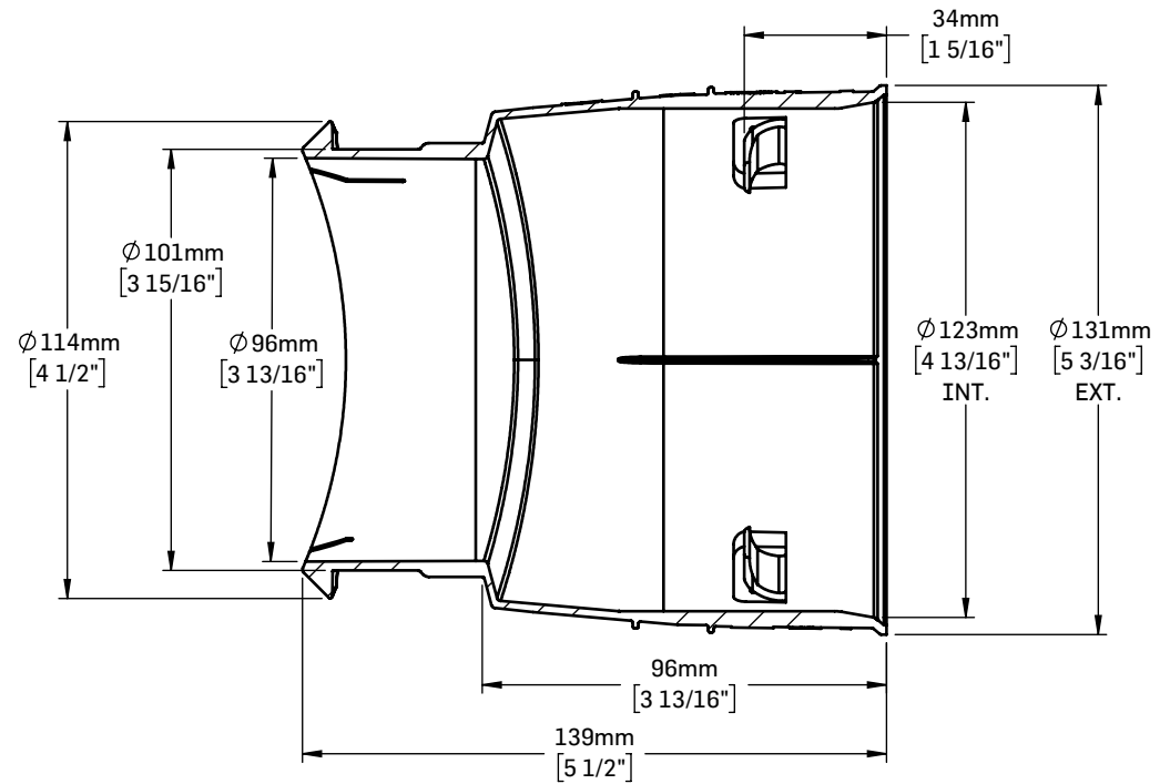
COUPE A-A
