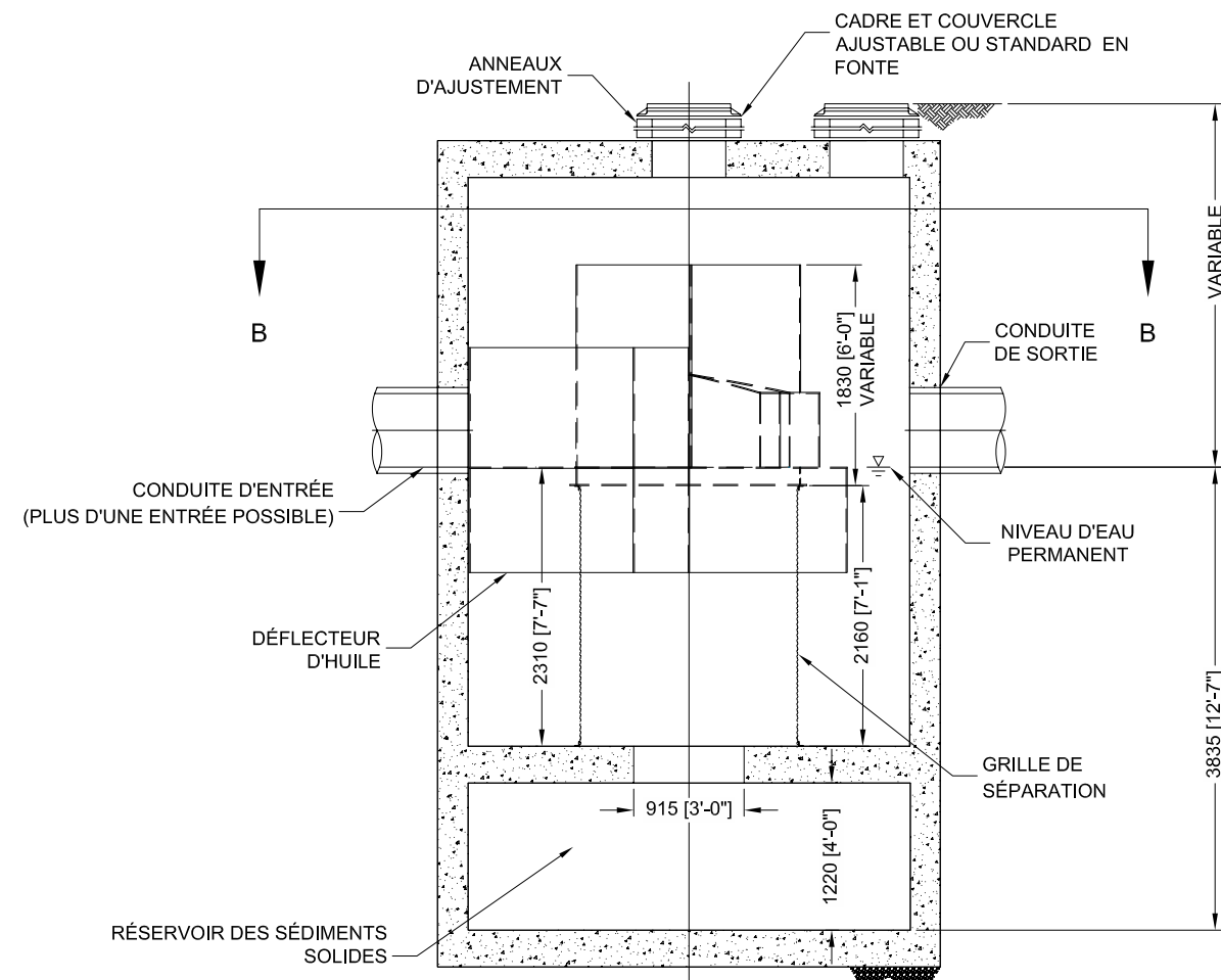
COUPE A-A ÉCHELLE: AUCUNE
