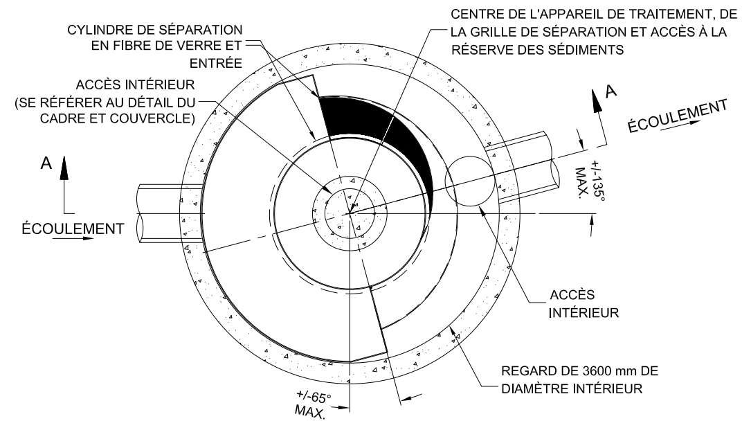
VUE EN PLAN B-B ÉCHELLE: AUCUNE
