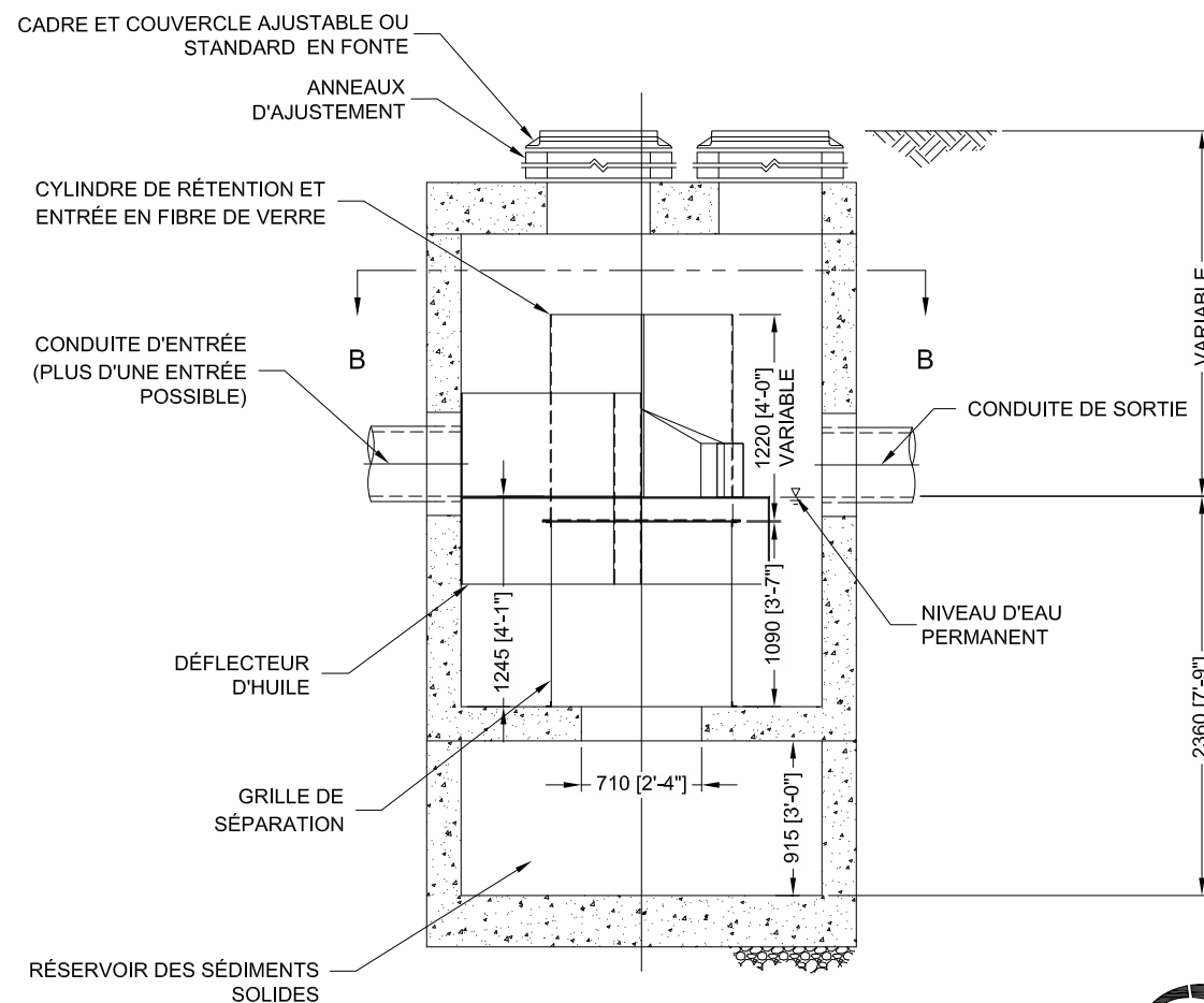
COUPE A-A
