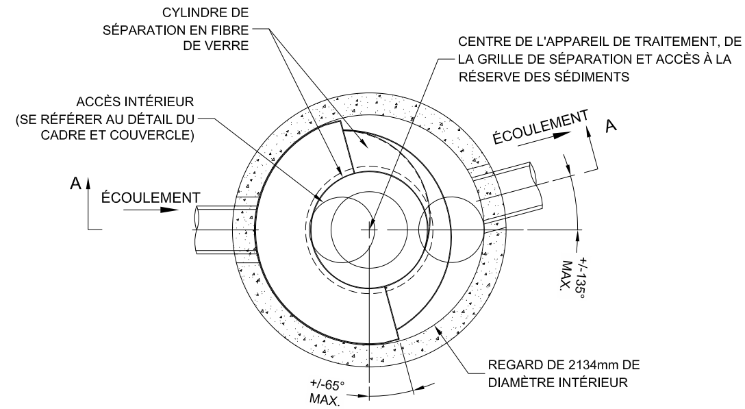
VUE EN PLAN B-B
