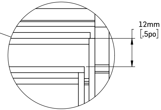
DÉTAIL A
