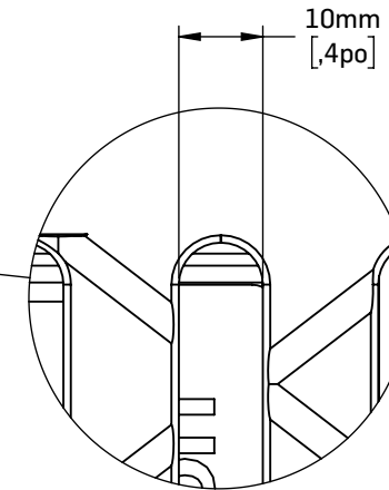
DÉTAIL A
