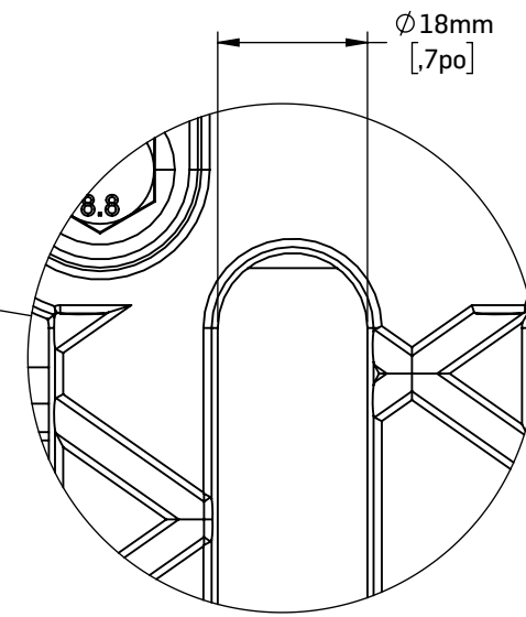
DÉTAIL A
