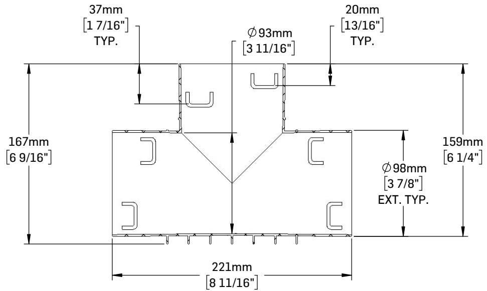
COUPE A-A
