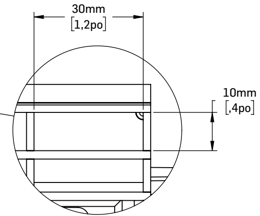
DÉTAIL A
