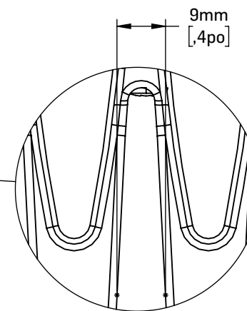
DÉTAIL A
