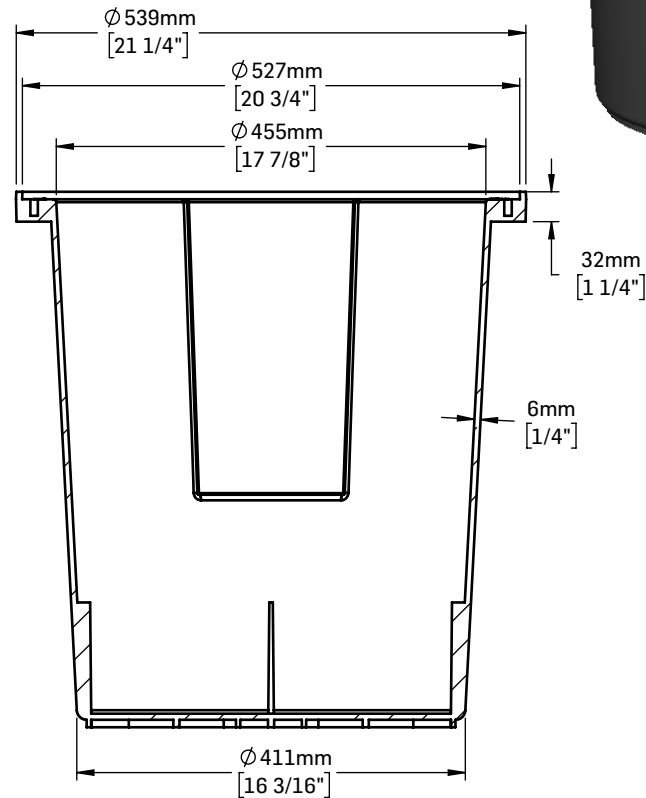
COUPE A-A
