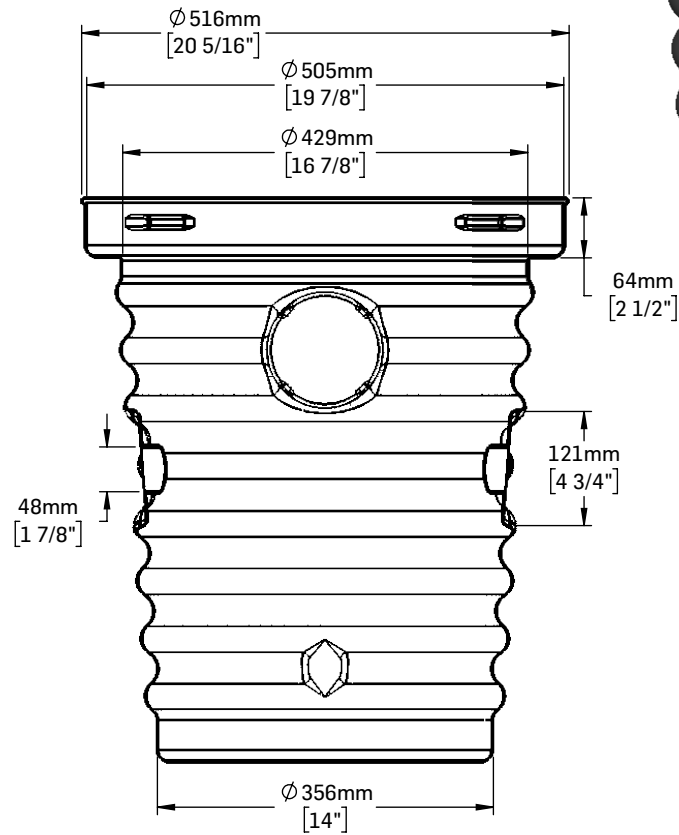
COUPE A-A
