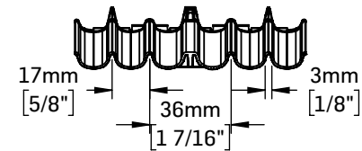
COUPE A-A
