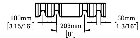
COUPE A-A
