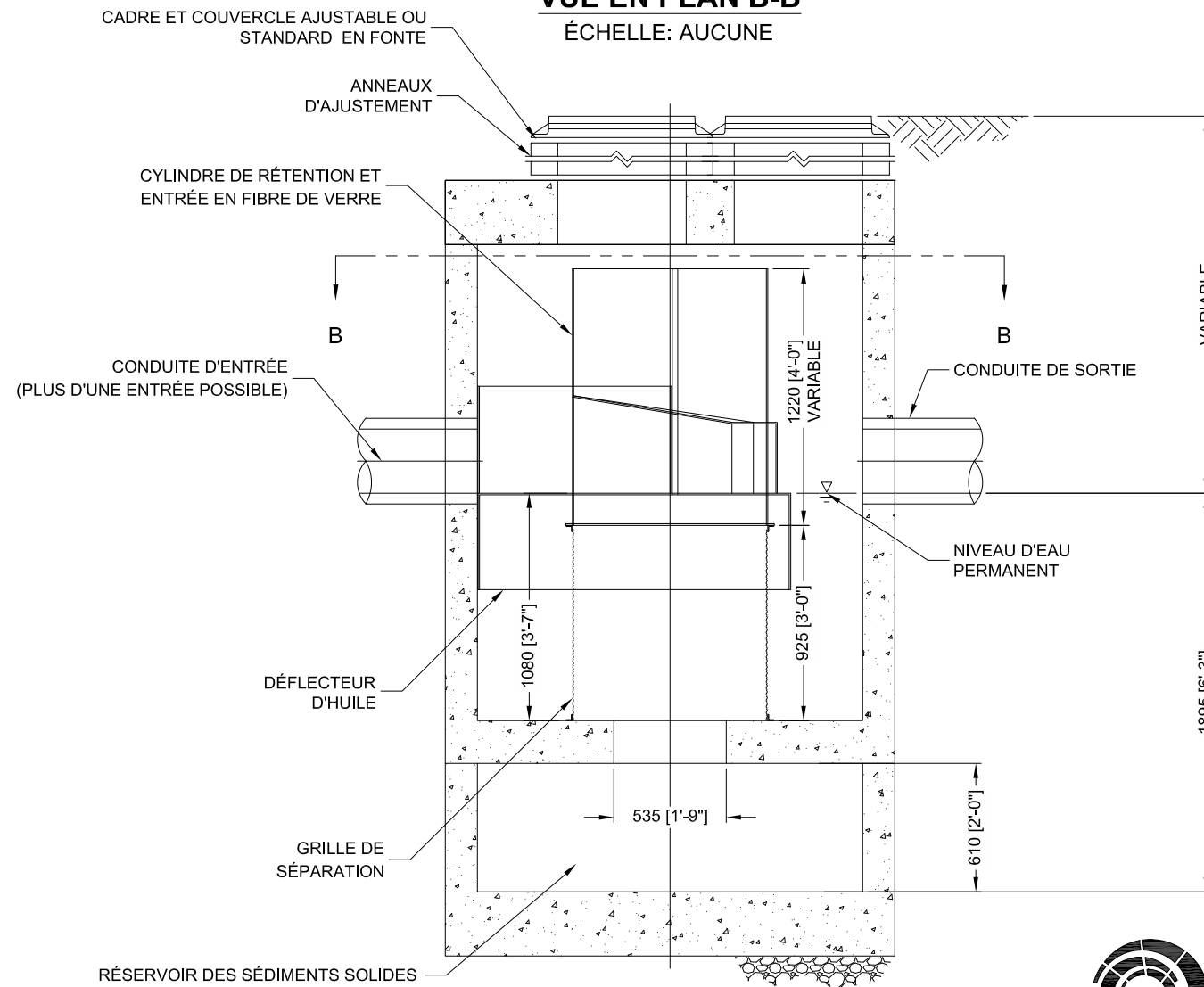
COUPE A-A ÉCHELLE: AUCUNE
