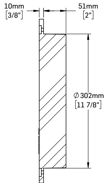
COUPE A-A
