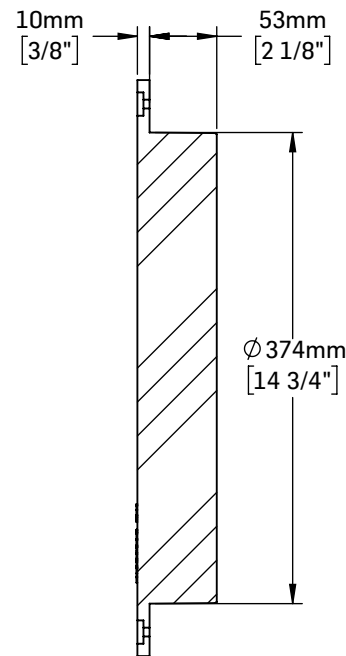
COUPE A-A
