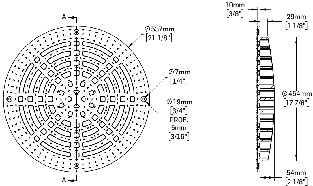
COUPE A-A
