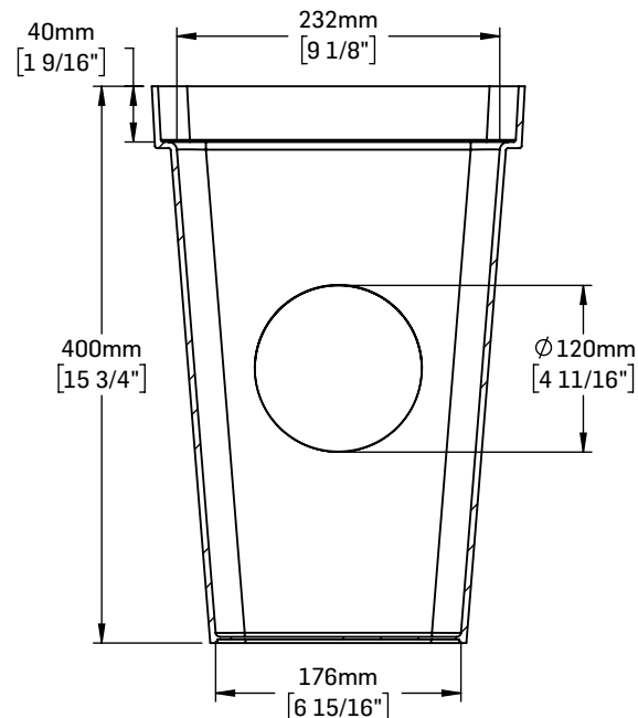
COUPE A-A
